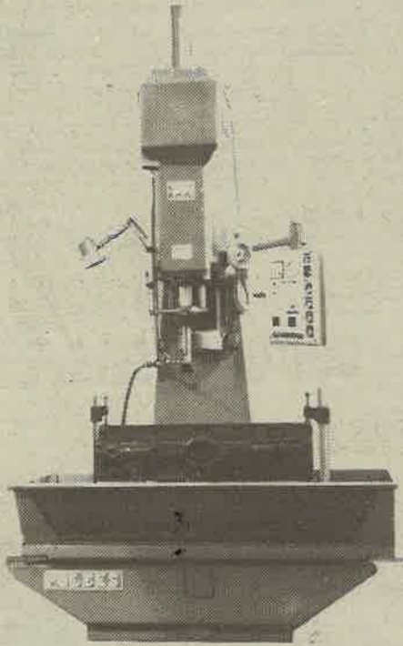
A. TIPI: Tam otomatik kendinden pasolu sabit hidrolikli (vertikal) Honlama makinesi strok 600 mm
